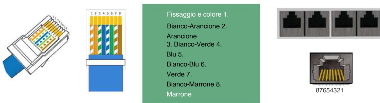
Figura 2-2 Definizione dell'interfaccia CAN, RS485, OUT, IN
