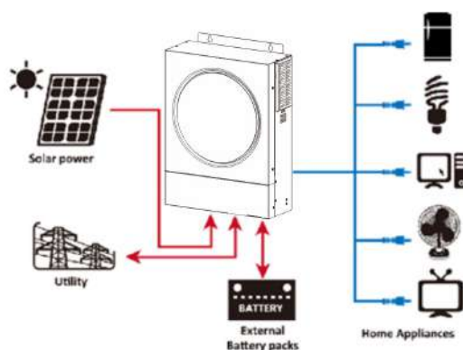
Figura 1 Panoramica Sistema FV ibrido base
